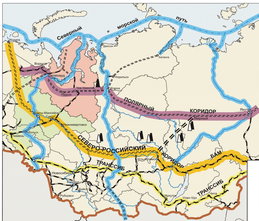
Рис. 1. Перспективные широтные транспортные коридоры Азиатской России первой половины XXI в.
